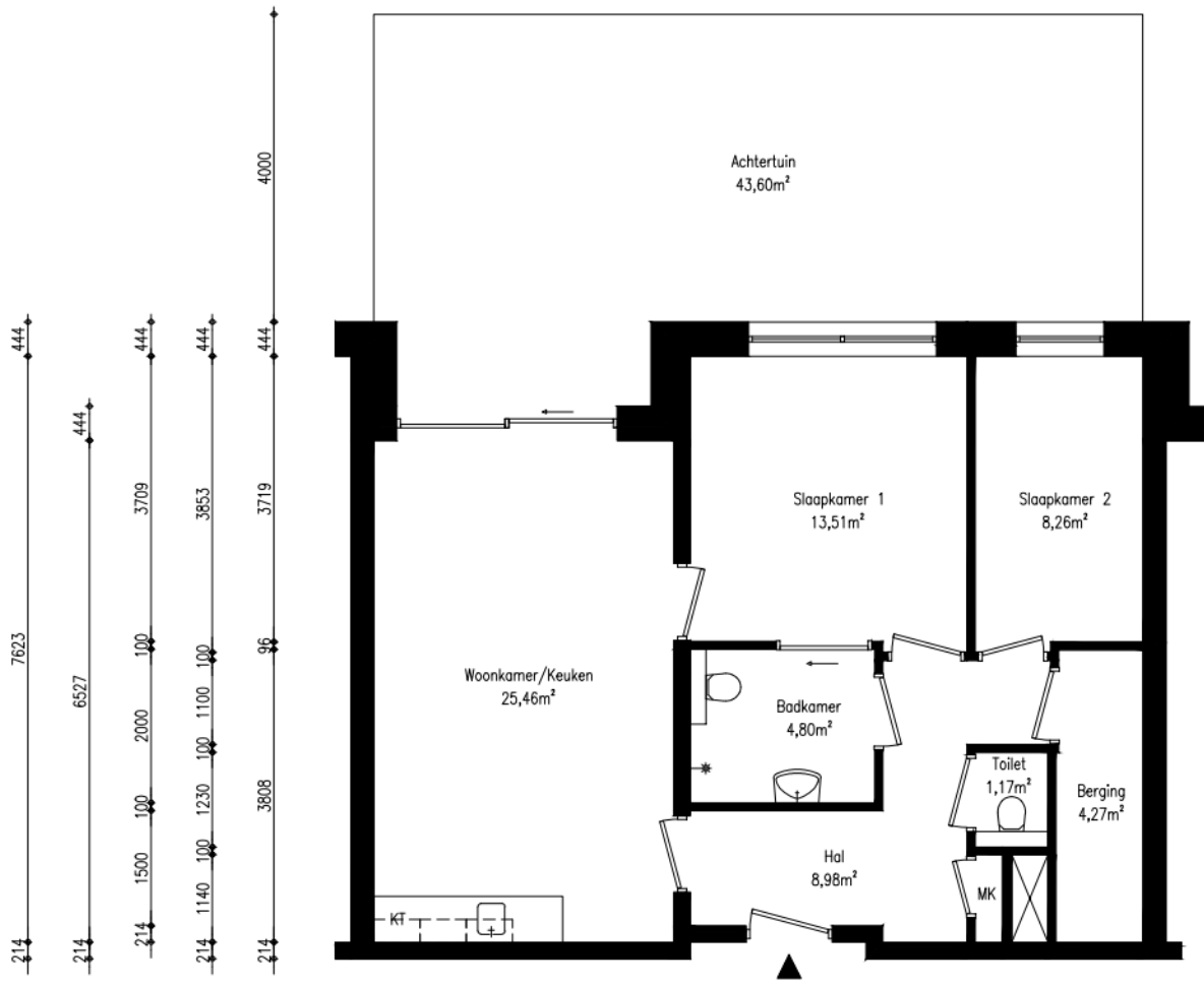
Begane grond
