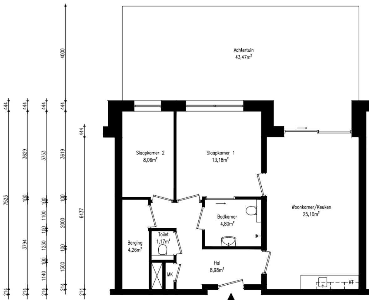
Begane grond
