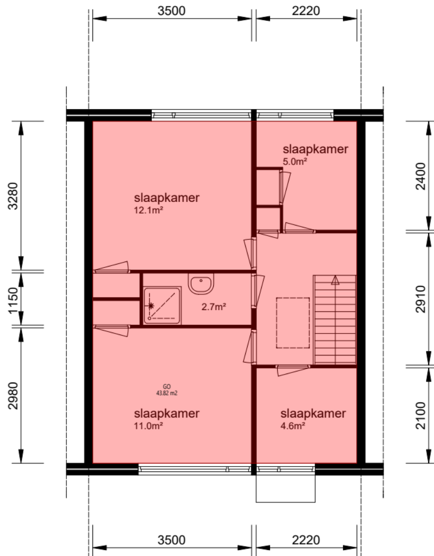
Verdieping_1e
