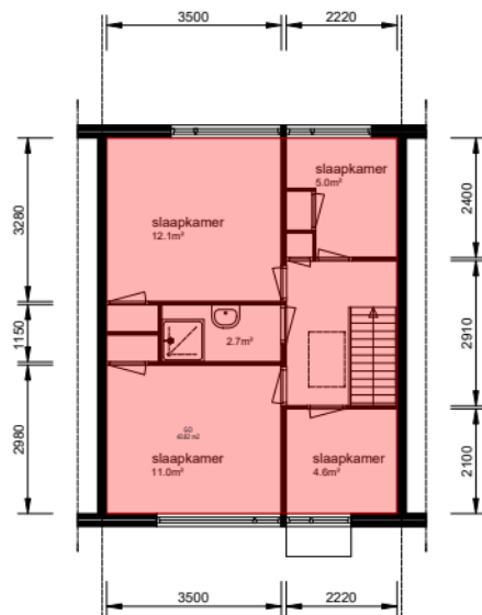
Verdieping_1e
