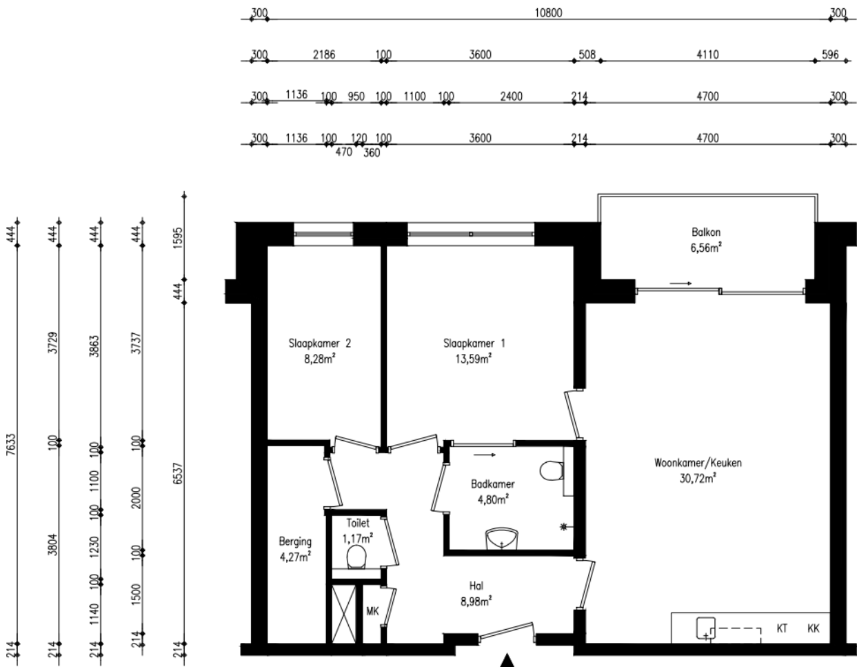
1e verdieping
