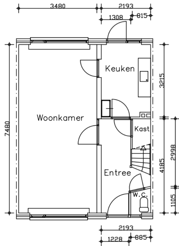
Beganegrond
