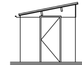
Voorgevel
