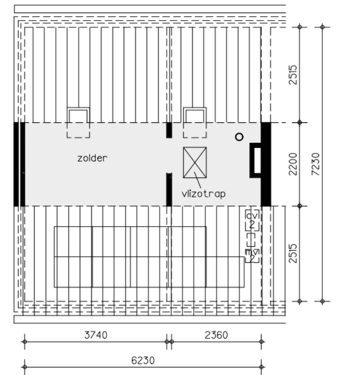
- 2e VERDIEPING -
