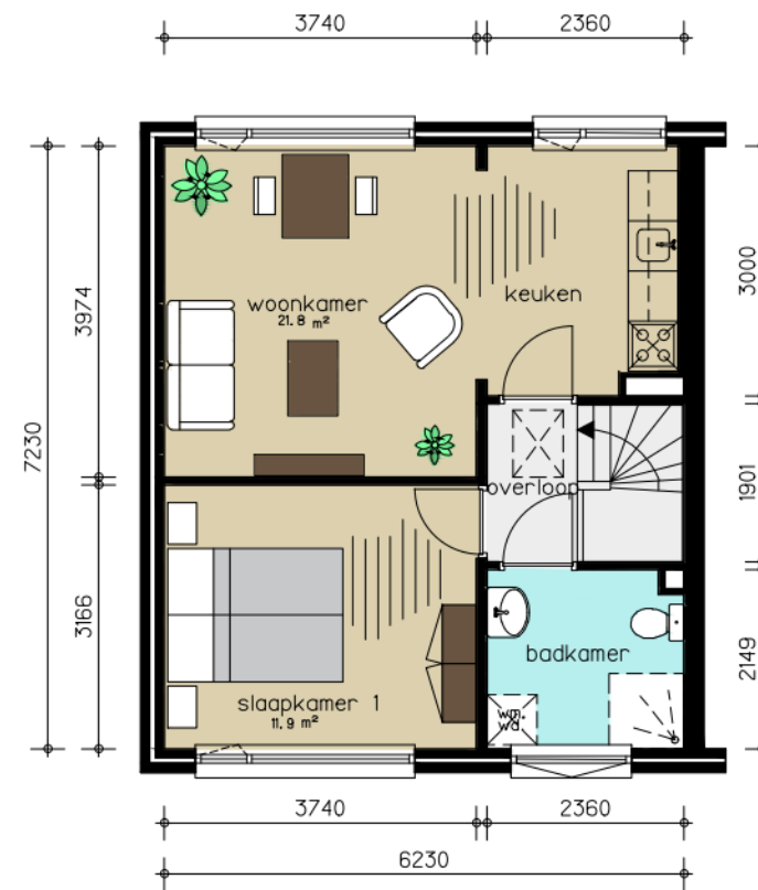
- 1e VERDIEPING -
