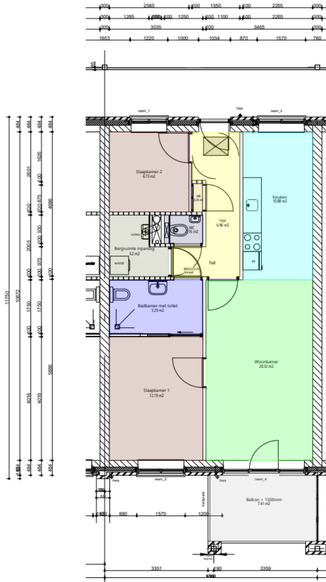
Verdieping_1e
