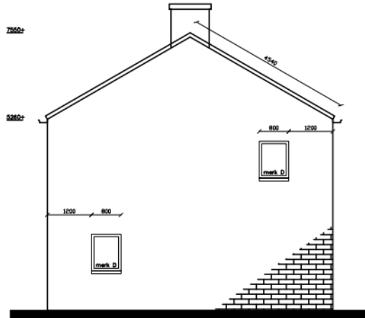
Kopgevel
