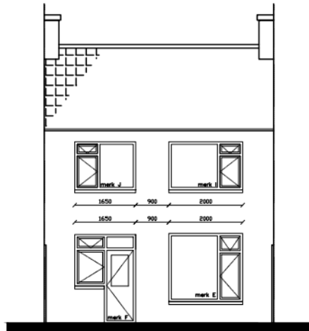
Achtergevels
