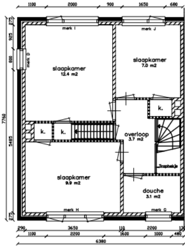
Verdieping
