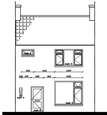
Voorgevels
