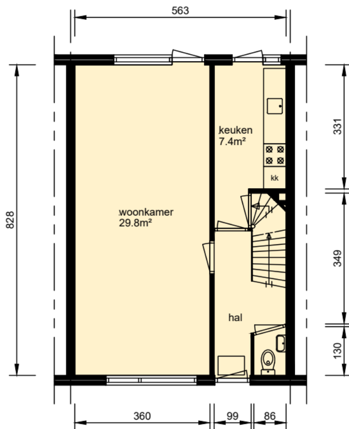
begane grond
