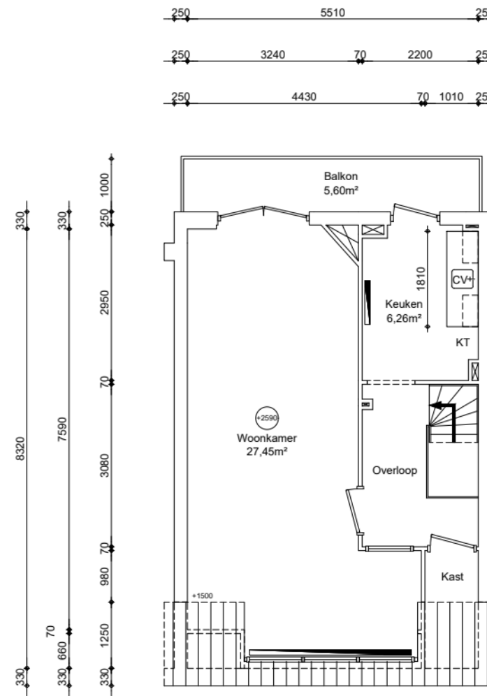
2e verdieping GO wonen 42,80m²
