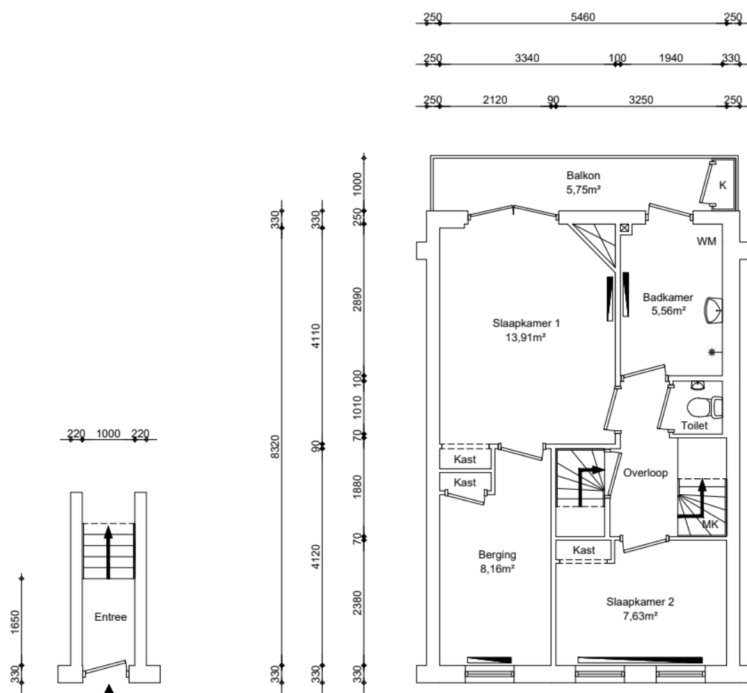
1e verdieping GO wonen 44,98m²
