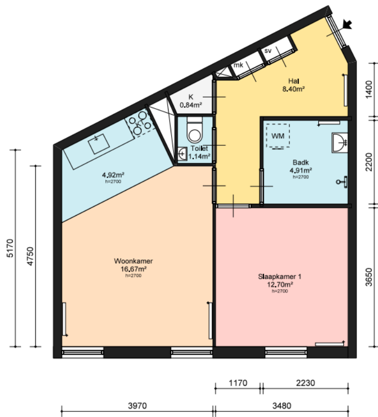
1e Verdieping
