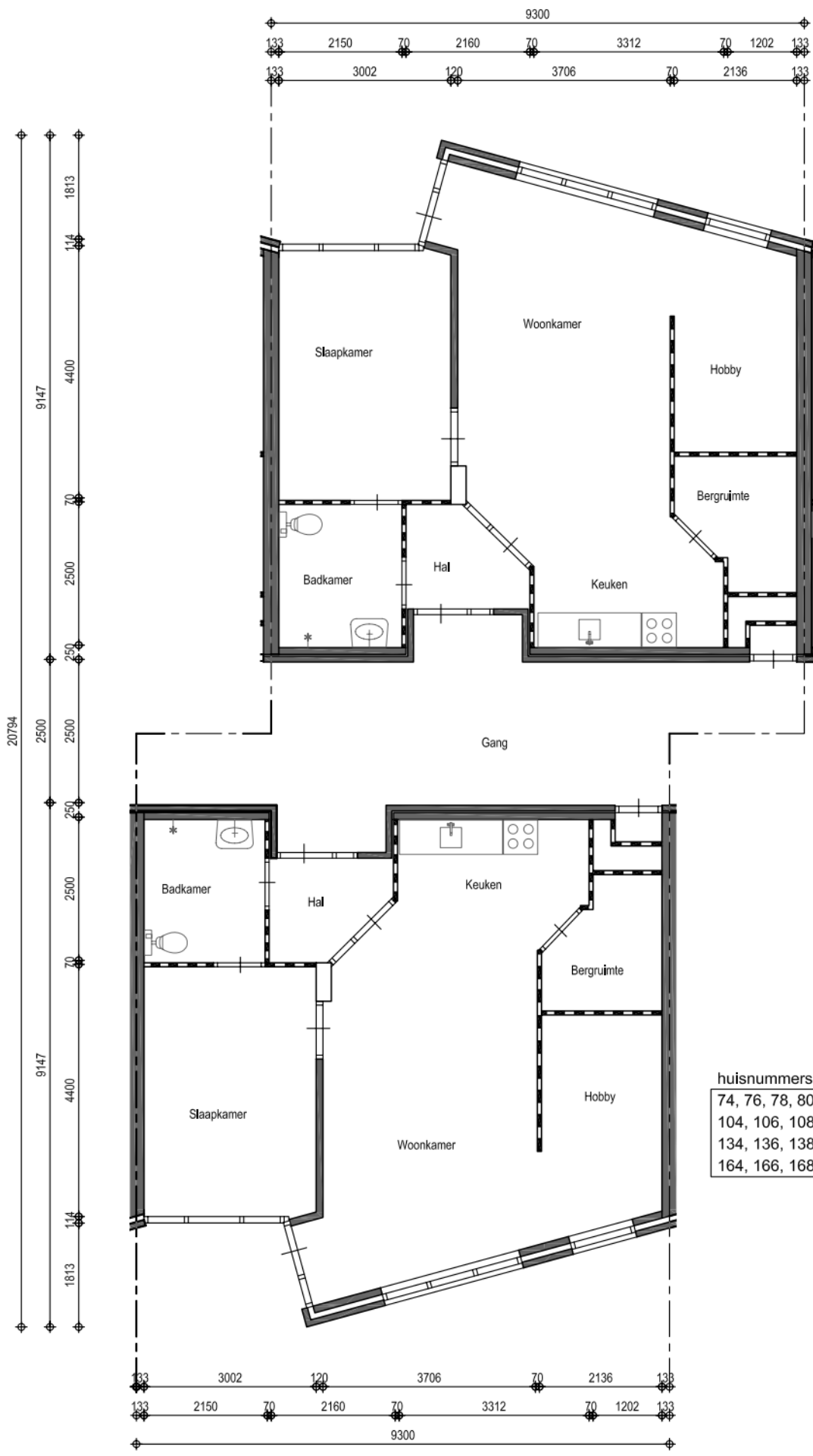
complex 078 - "Internos" Rembrandtlaan Plattegrond
