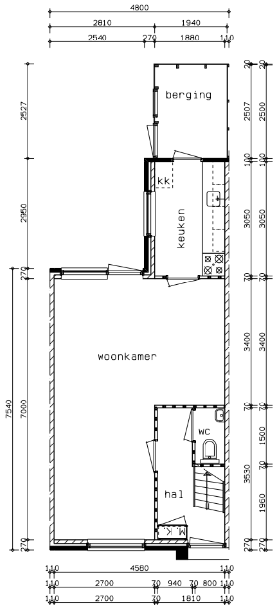
BEGANE GROND
