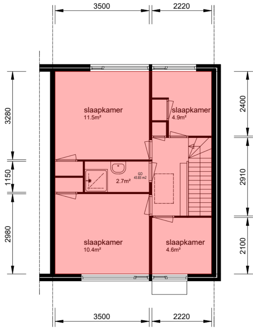
Verdieping_1e
