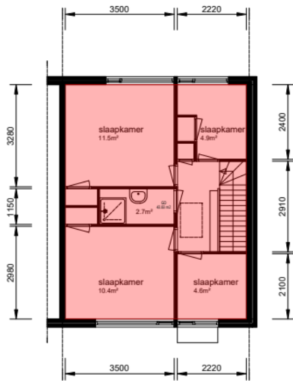
Verdieping_1e
