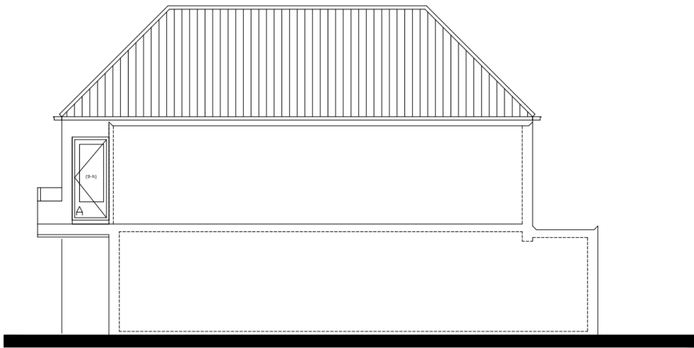
RECHTER ZIJGEVEL
