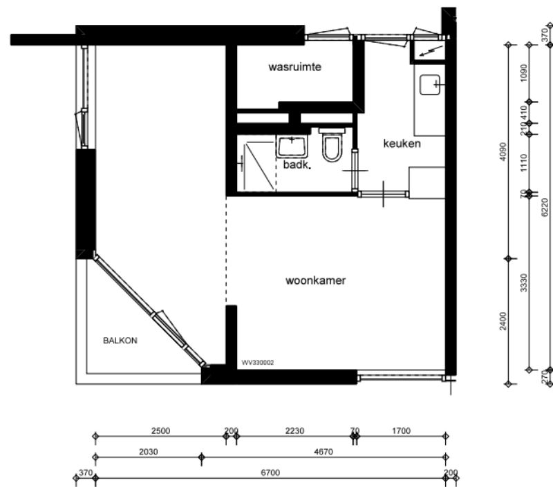
VERDIEPING
