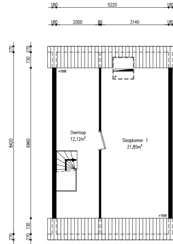
2e verdieping
