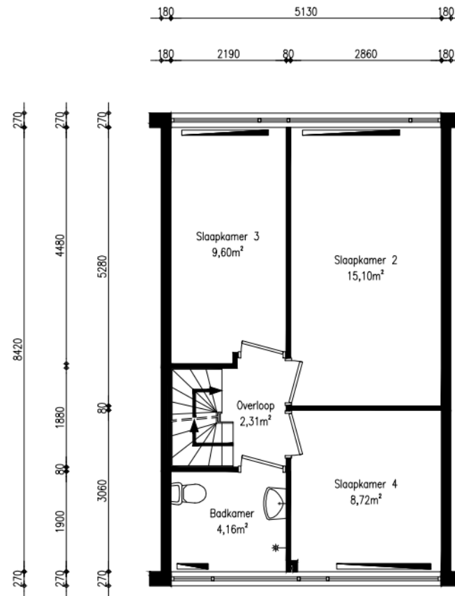
1e verdieping
