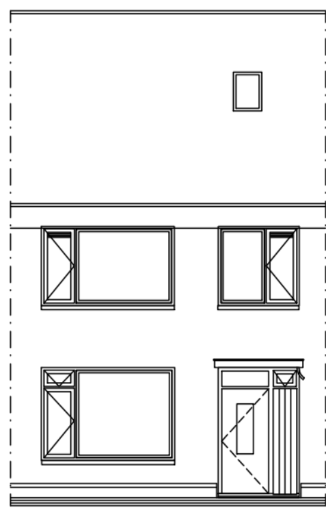
Voorgevel
