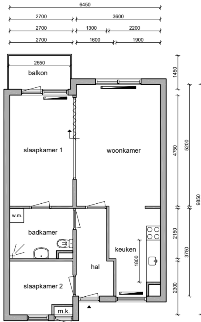
Appartement begane grond
