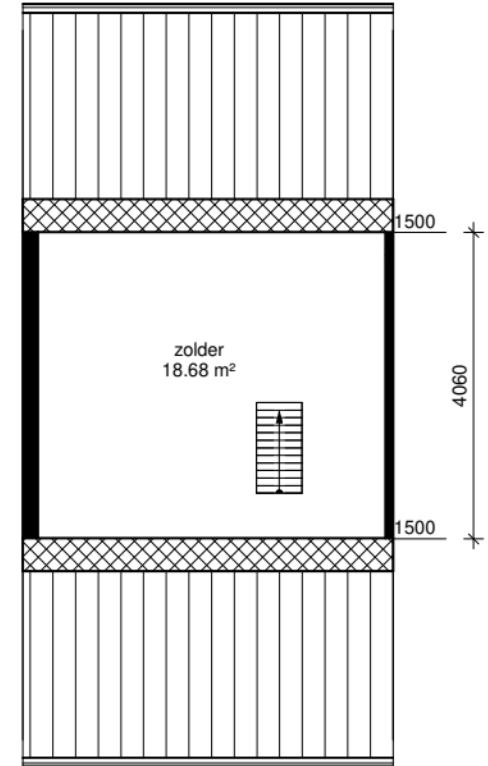
tweede verdieping
