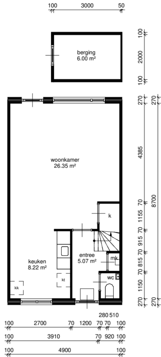
begane grond
