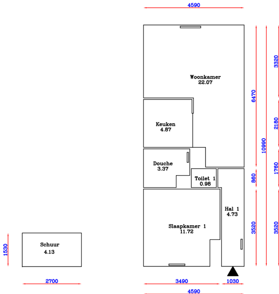
Begane grond
