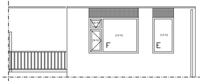
ACHTERGEVEL
