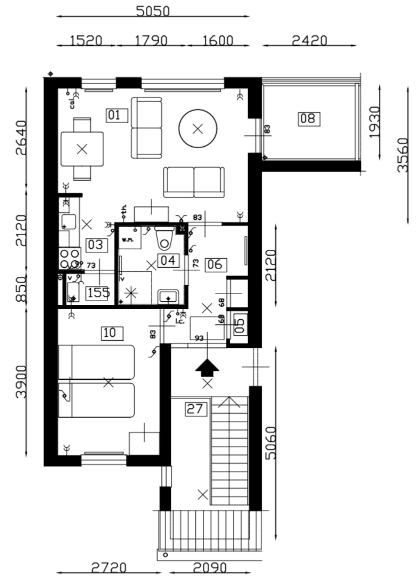
PLATTEGROND
