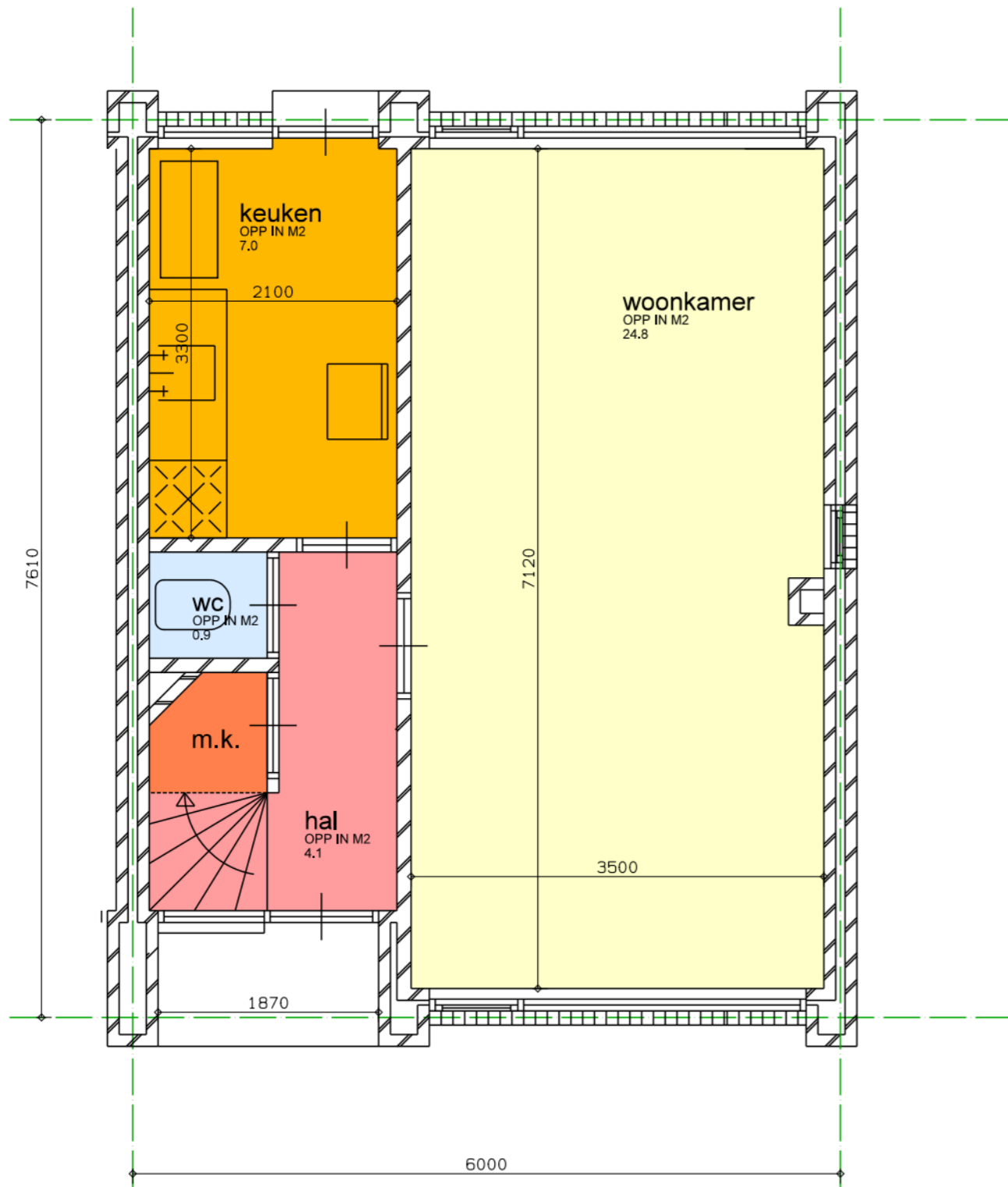
begane grond
