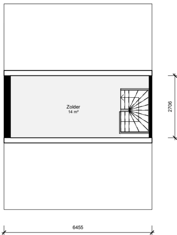
02 Tweede verdieping
