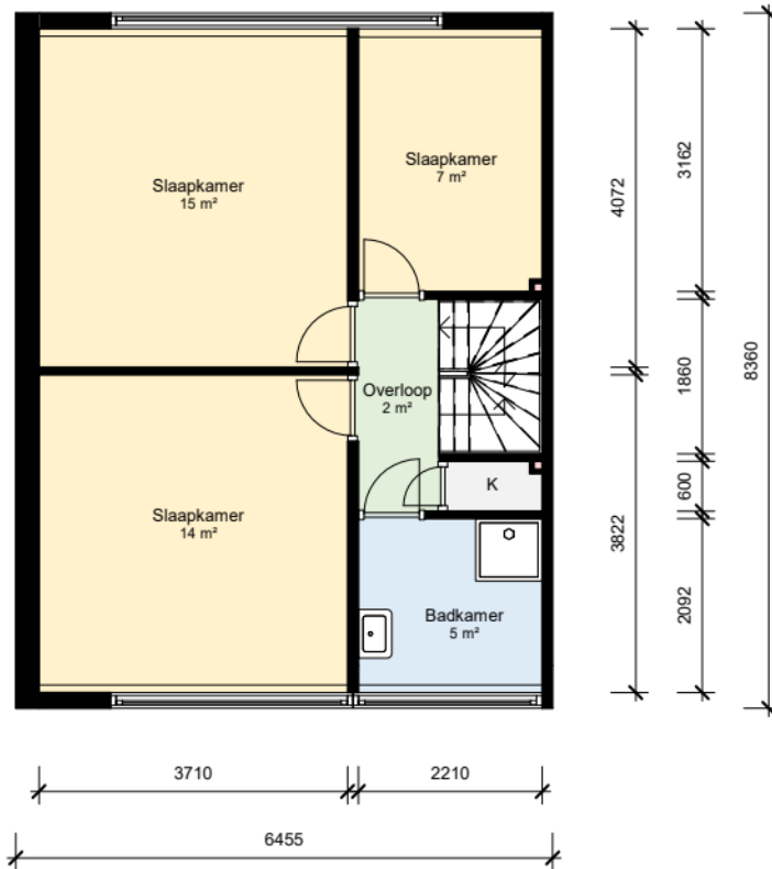
01 Eerste verdieping
