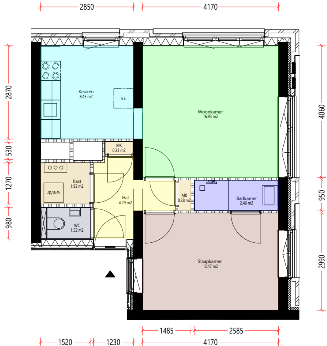
Verdieping_1e
