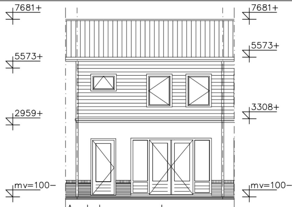
Achtergevel
