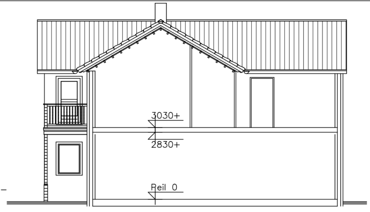
Doorsnede
