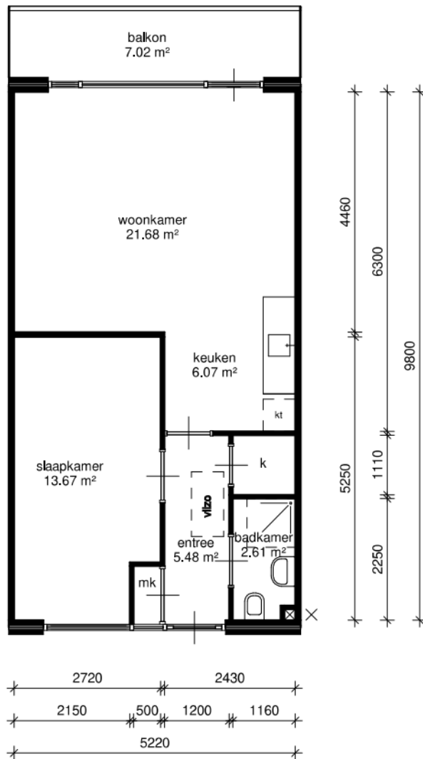
tweede verdieping
