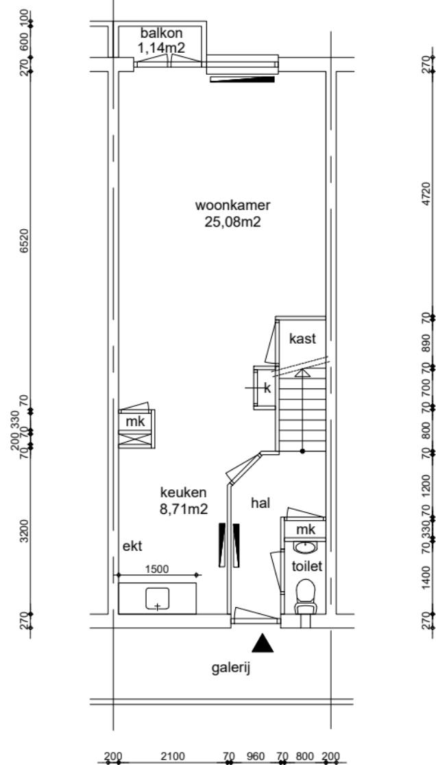
Begane grond GO wonen 41,84m²
