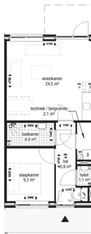
Begane grond
