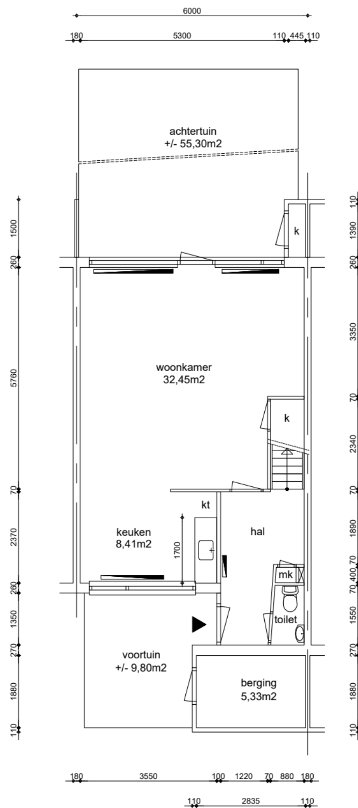
Begane grond GO wonen 51,22m 2
