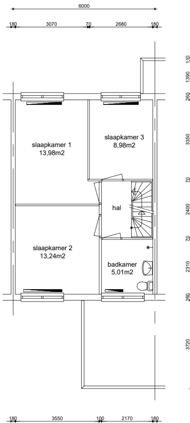
1e verdieping GO wonen 42,72m 2
