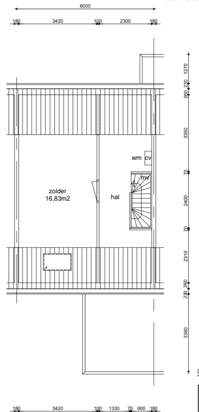
2e verdieping GO wonen 28,63m 2
