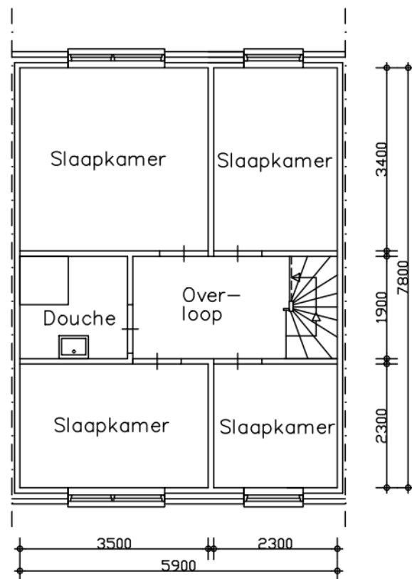
Verdieping
