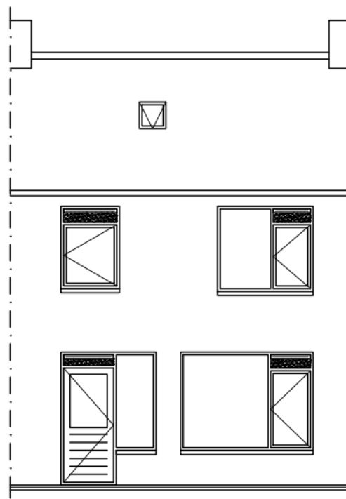
Achtergevel
