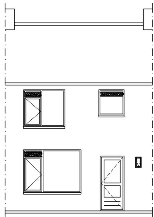
Voorgevel
