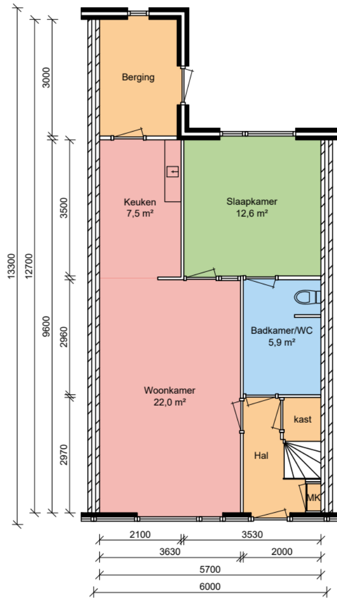
Begane grond
