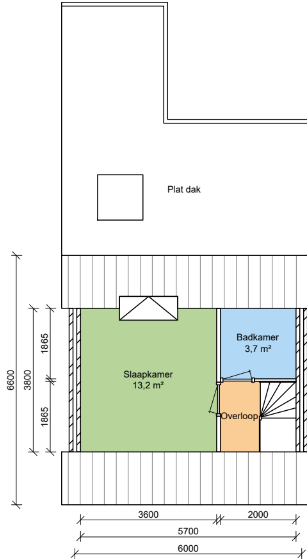
Verdieping
