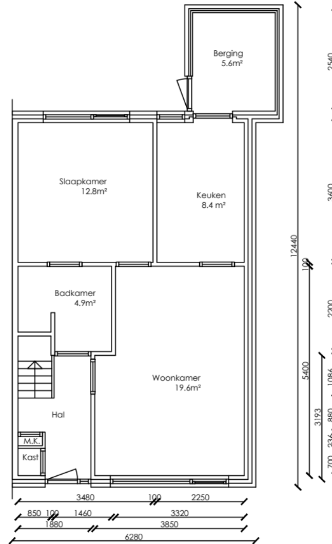
Begane grond
