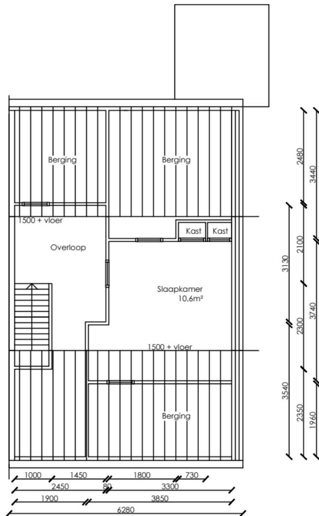
Verdieping
