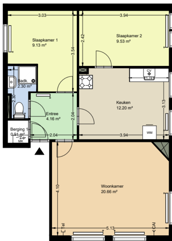
2e verdieping
