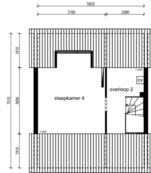
2e verdieping
