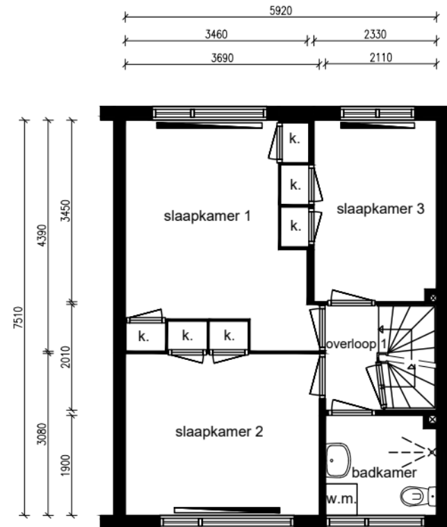
1e verdieping
