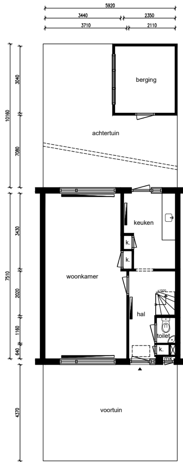
Begane grond
