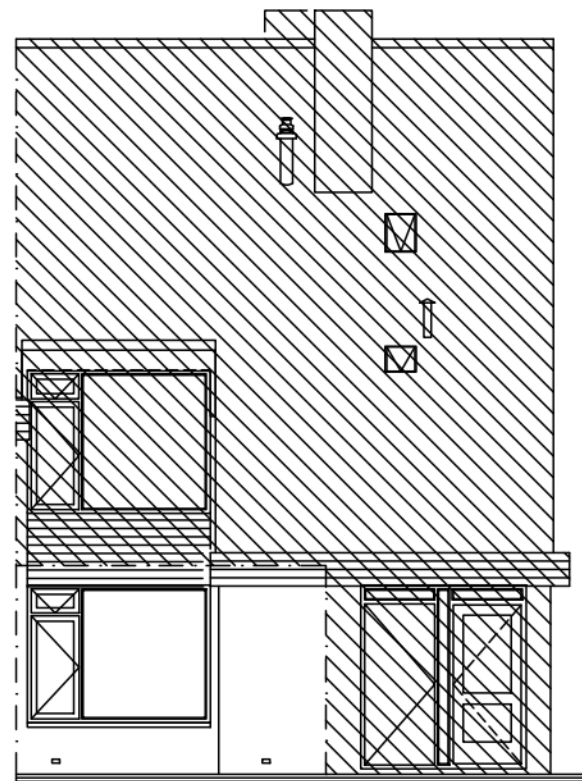
Voorgevel
