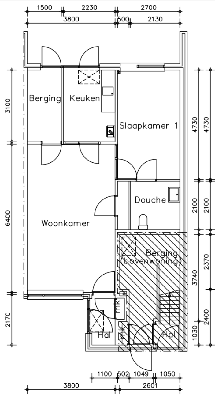
Beganegrond
