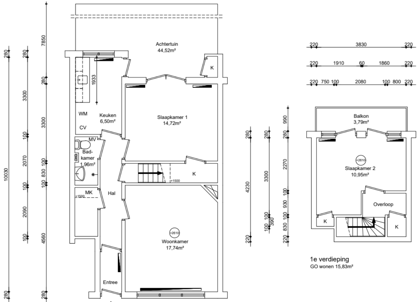
Begane grond GO wonen 50,72m 2
