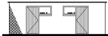
VOORGEVEL schuur
