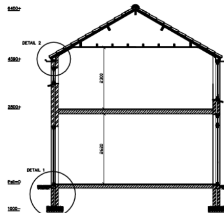
DOORSNEDE schaal 1:50
