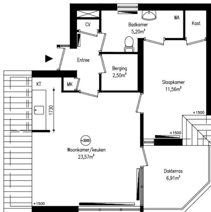
2e verdieping
