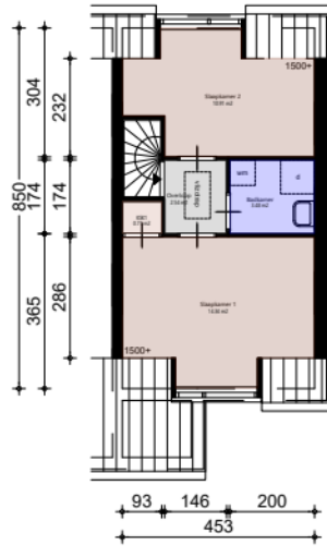
Verdieping_1e
