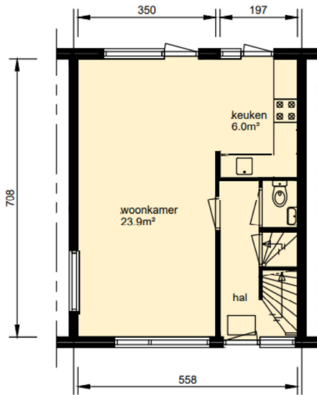
begane grond
