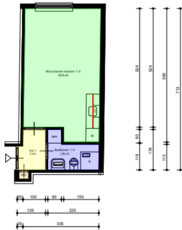
Begane grond
