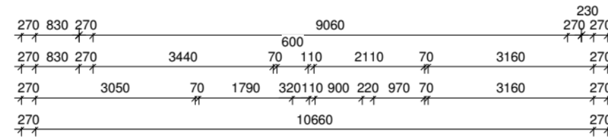
derde verdieping
