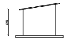
ZIJGEVEL
