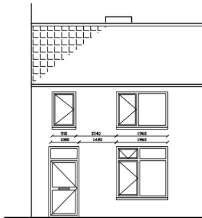
VOORGEVELS
