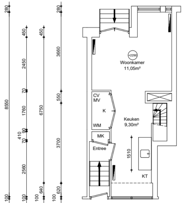
Begane grond GO wonen 24,74m 2
