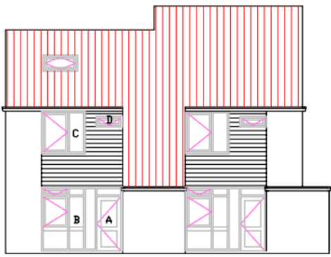
Voorgevel
