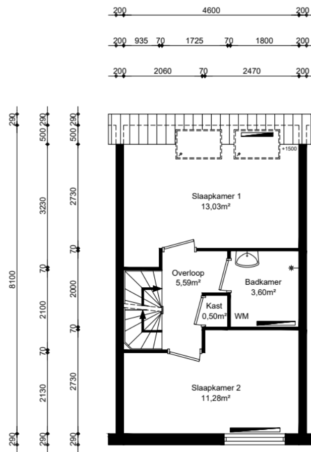
1e verdieping
