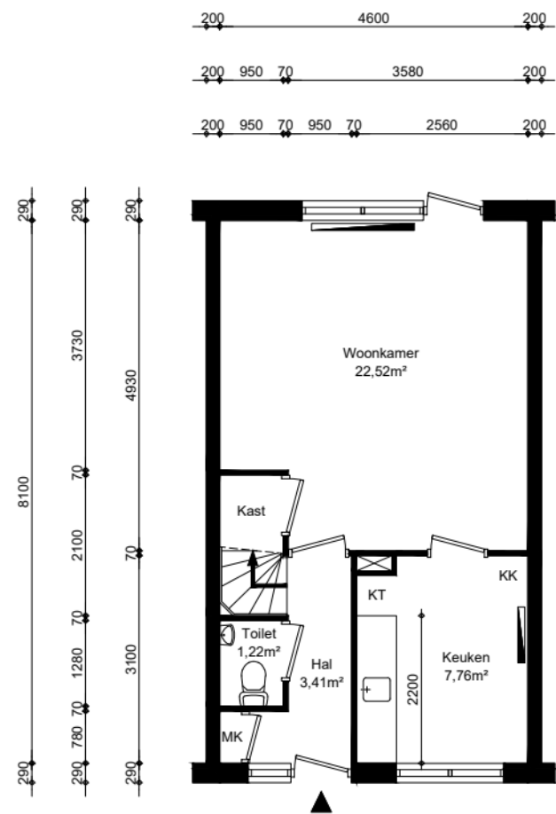
Begane grond
