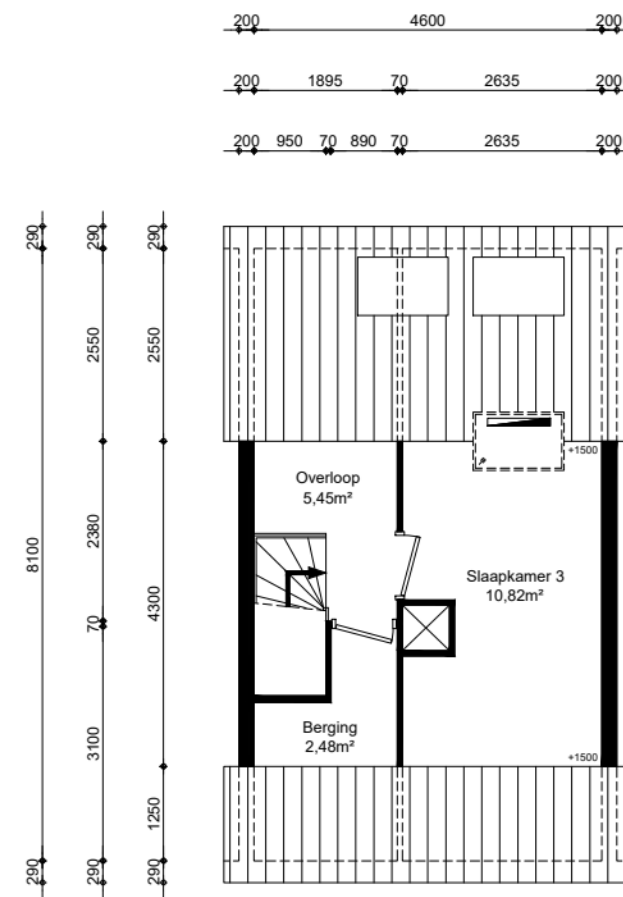
2e verdieping
