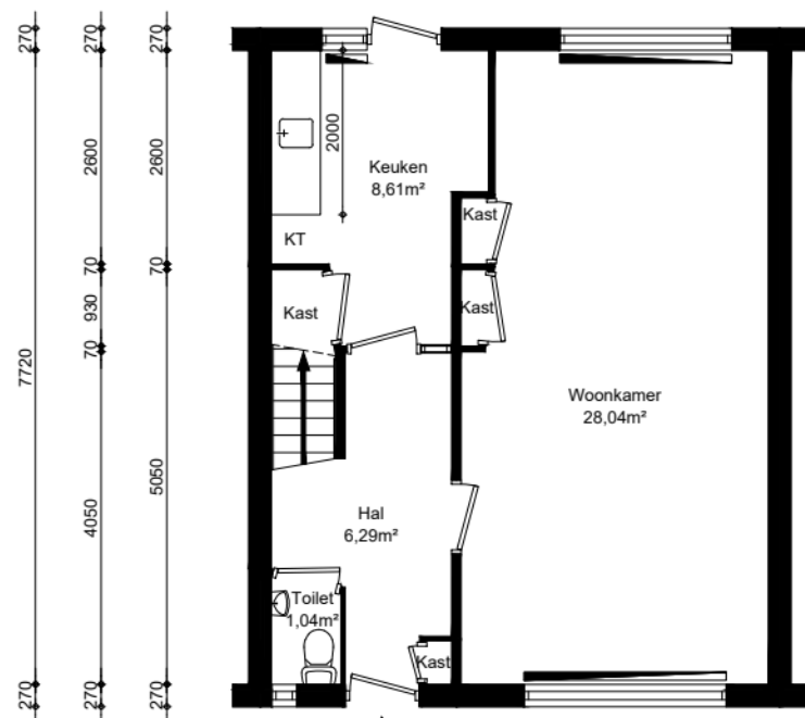
Begane grond
