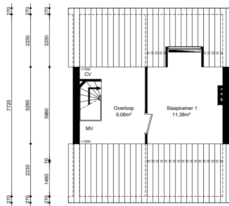
2e verdieping
