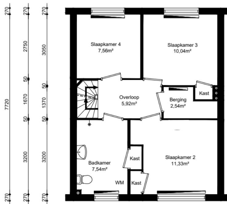
1e verdieping
