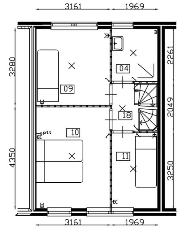
EERSTE VERDIEPING
