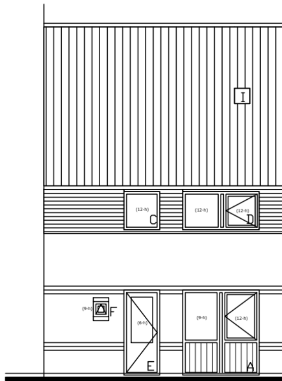
ACHTERGEVEL
